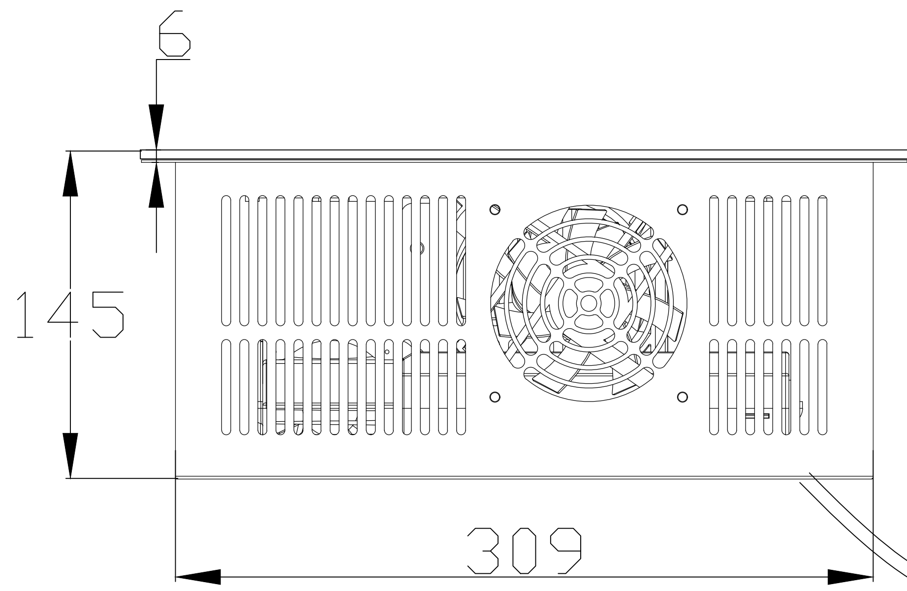
仰视图
